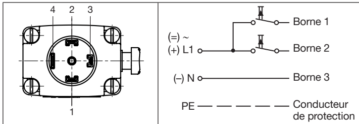
Fig. 8 : Schéma électrique
