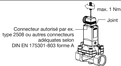
Fig. 7 : Raccordement électrique du connecteur
